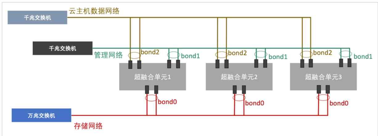
图 3: 超融合-三节点网络拓扑
